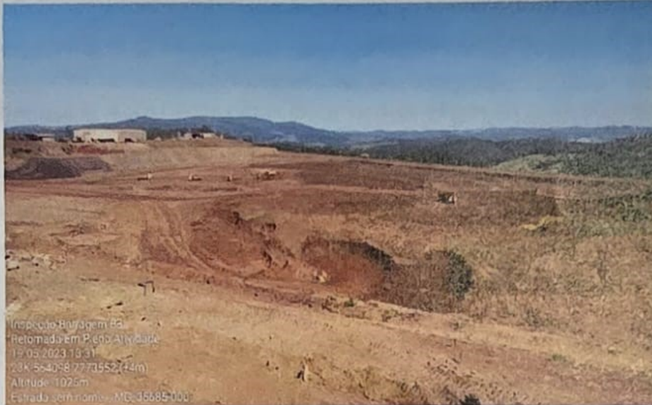
Escavação realizada por conjuntos escavadeiras e caminhões basculantes.
